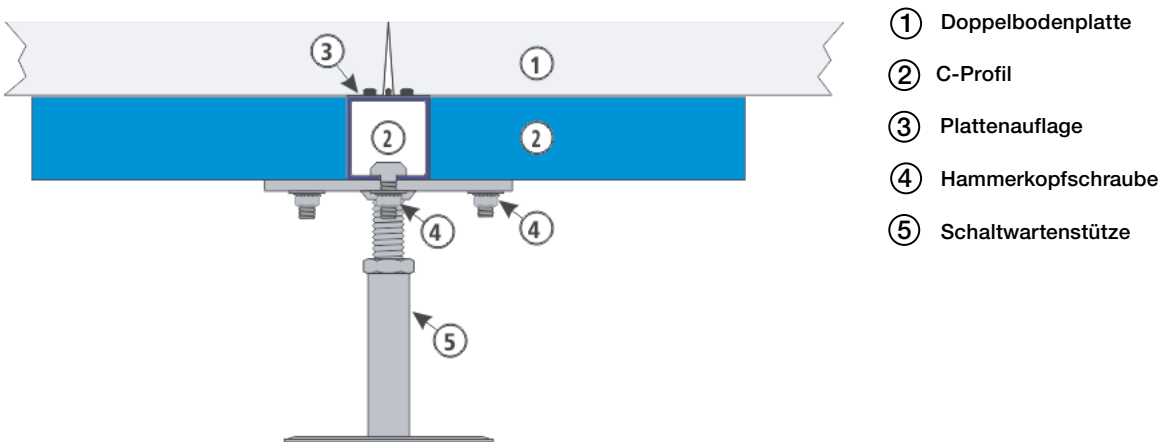
Plattenauflage
